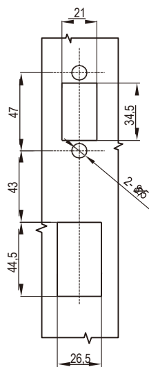
Монтажное отверстие
