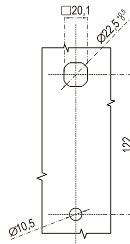
Монтажное отверстие
