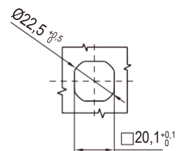
Монтажное отверстие
