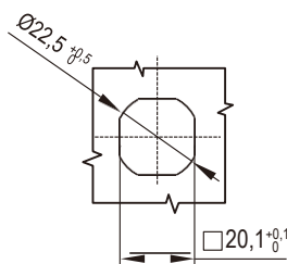
Монтажное отверстие
