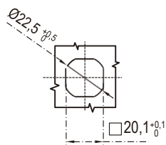
Монтажное отверстие
