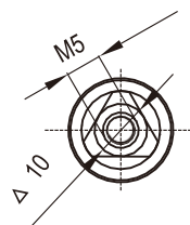
Трехгранник 10 мм с отверстием для винта М5
