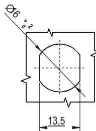
Монтажное отверстие
