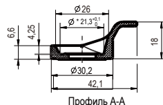
Профиль А-А
