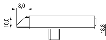
112 Исполнение под сварку-112
