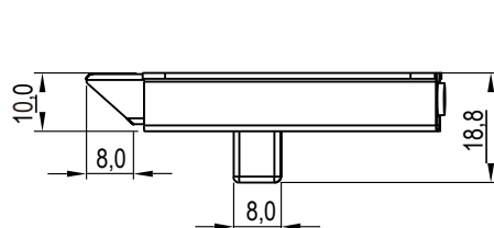
Исполнение с винтовым креплением-011
