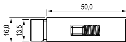
Исполнение с винтовым креплением-011
