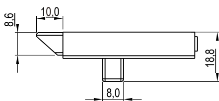
012 Исполнение под сварку-012
