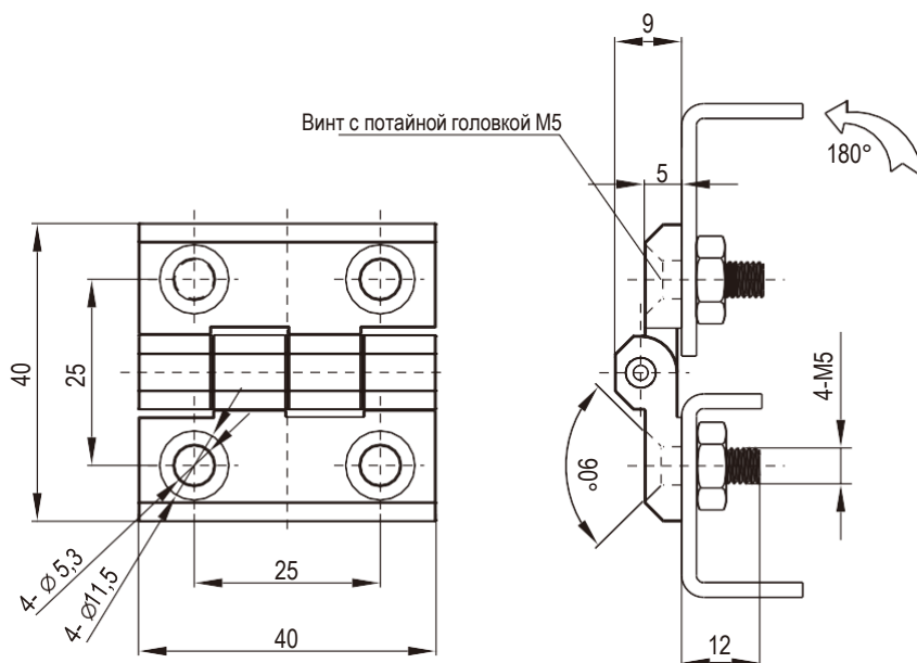
Винт с потайной головкой M5
