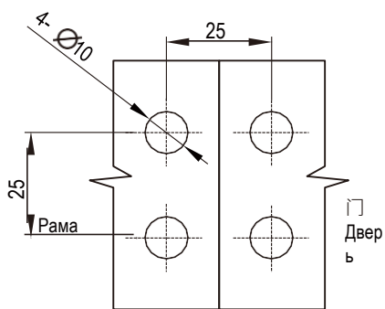
Монтажное отверстие
