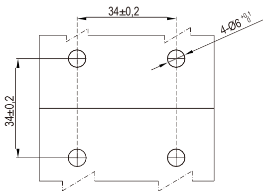
Монтажное отверстие
