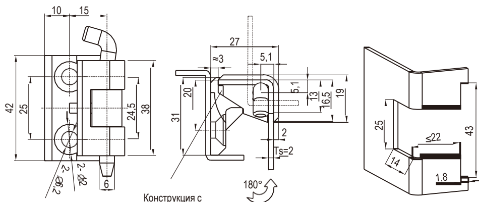
Конструкция с защитой от падения
