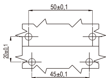
Монтажное отверстие
