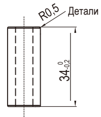
Исполнение В
