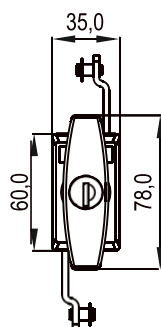
Штанговый механизм
