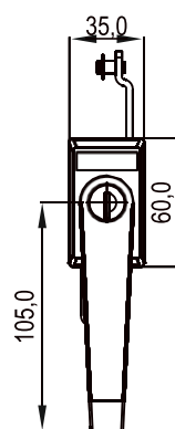
Л-образная ручка
